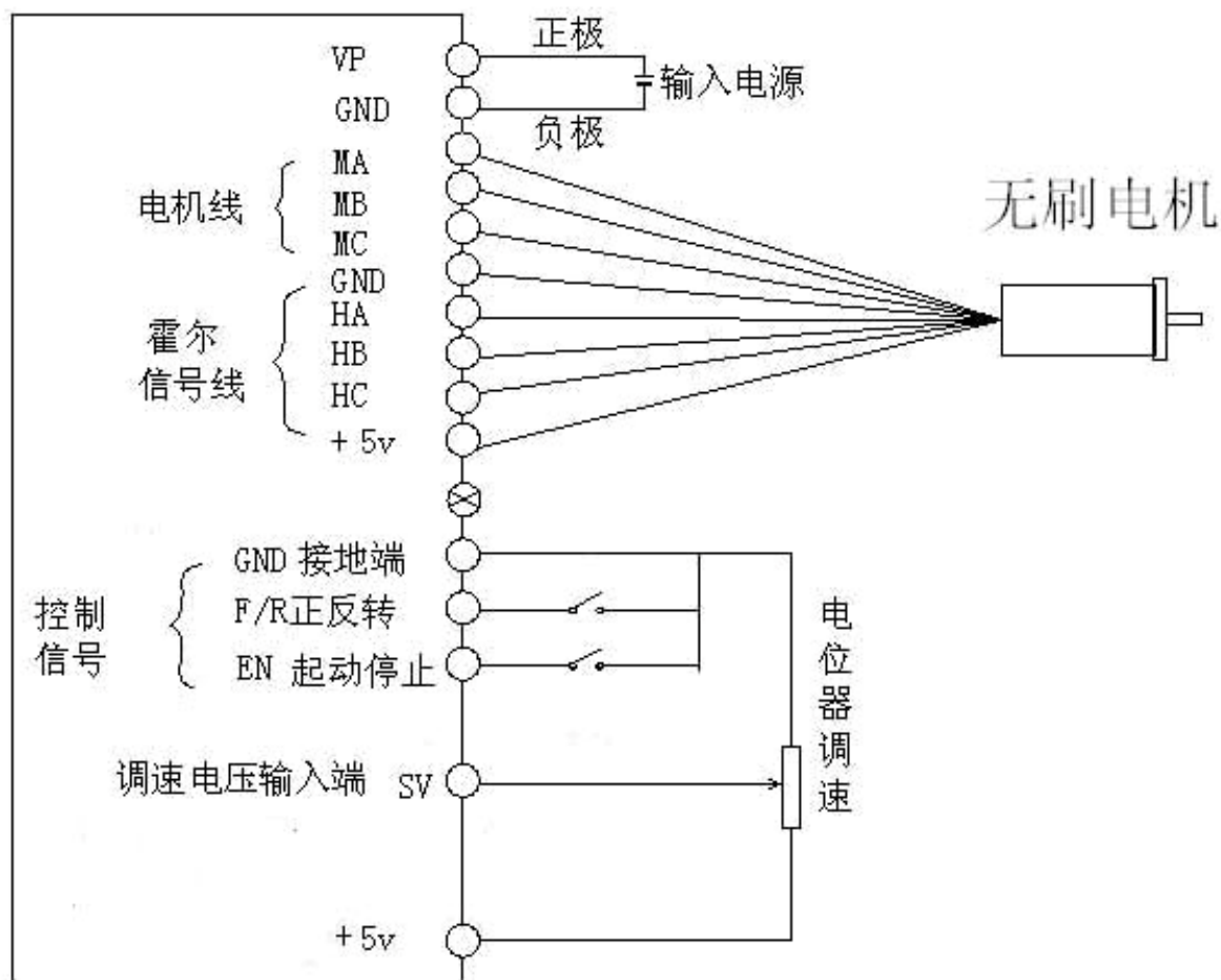
驱动器与无刷电机接线图
